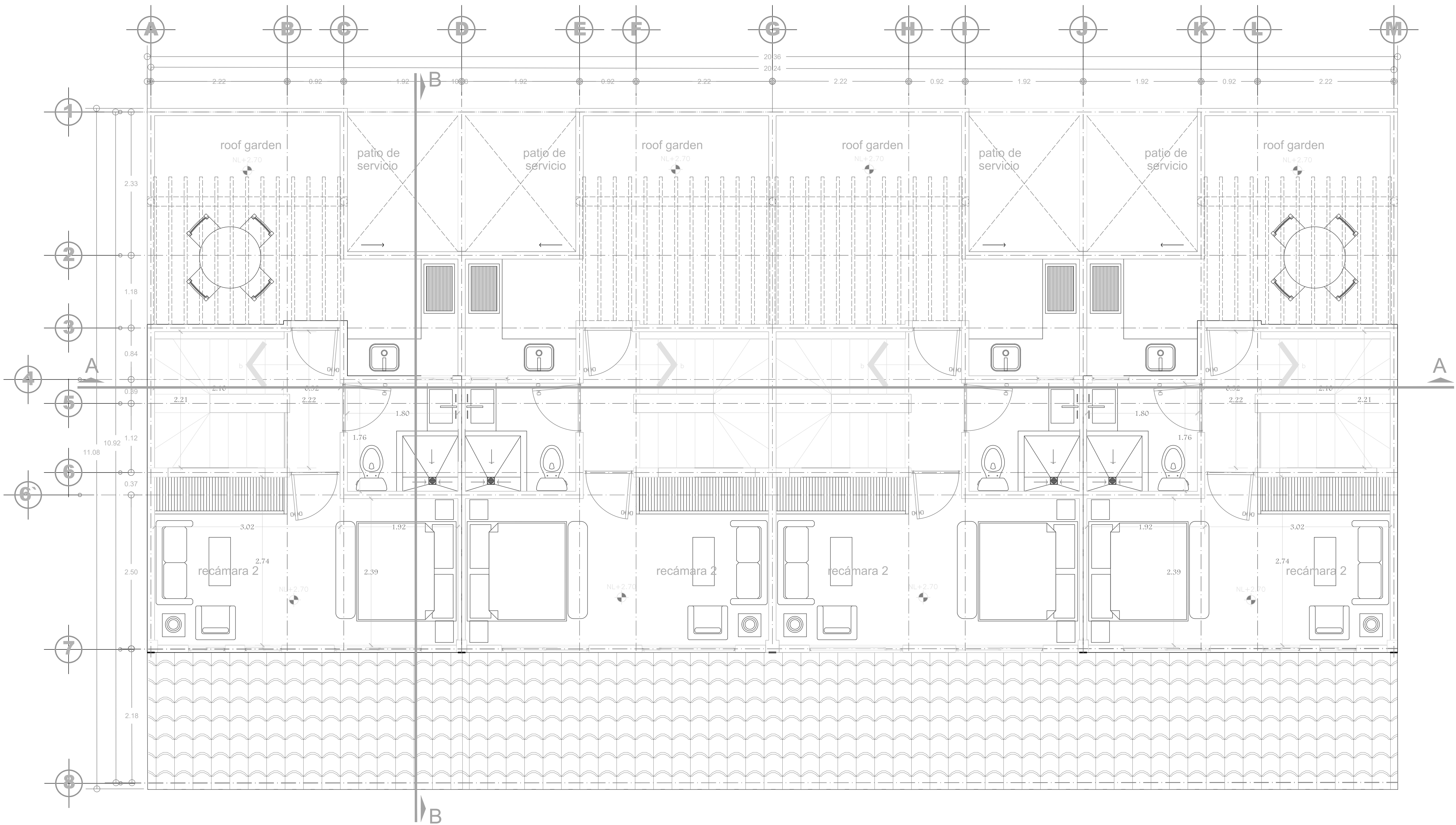
PLANTA ARQUITECTONICA 1er. NIVEL
