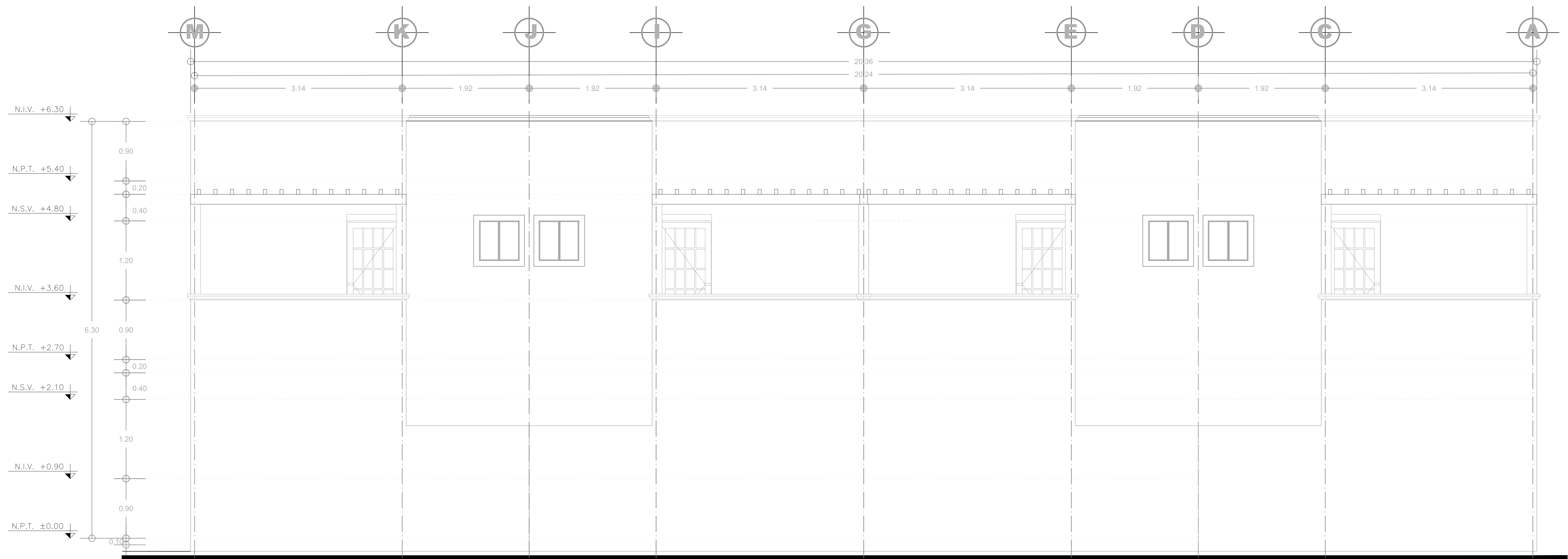
FACHADA POSTERIOR
