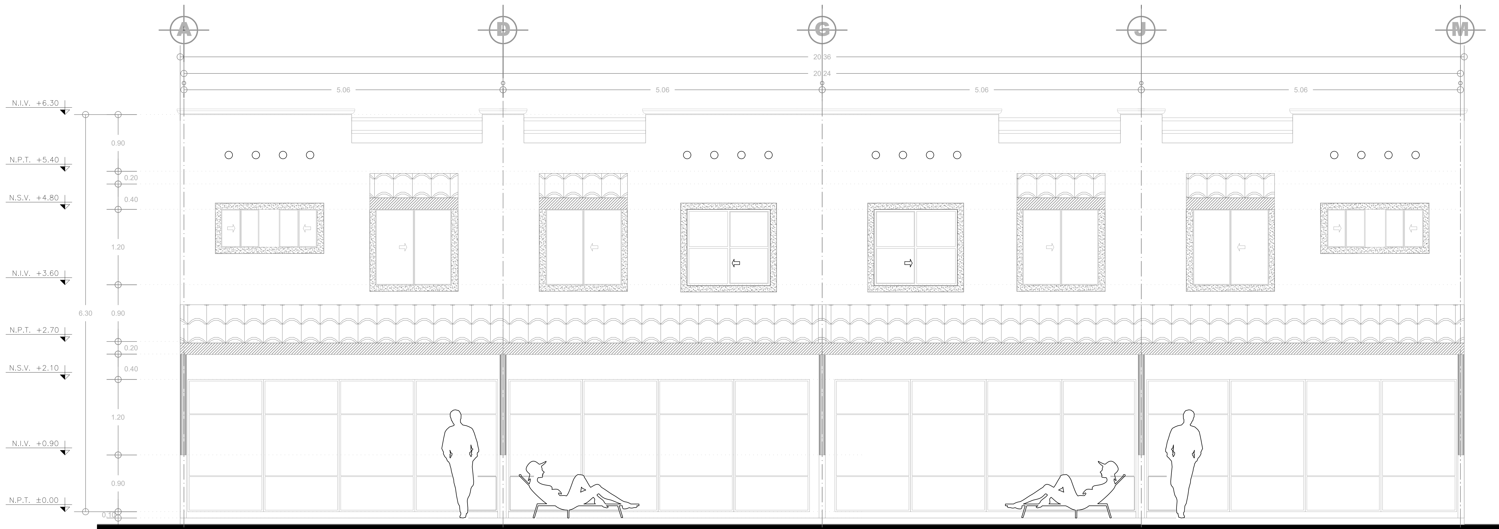
FACHADA FRONTAL
