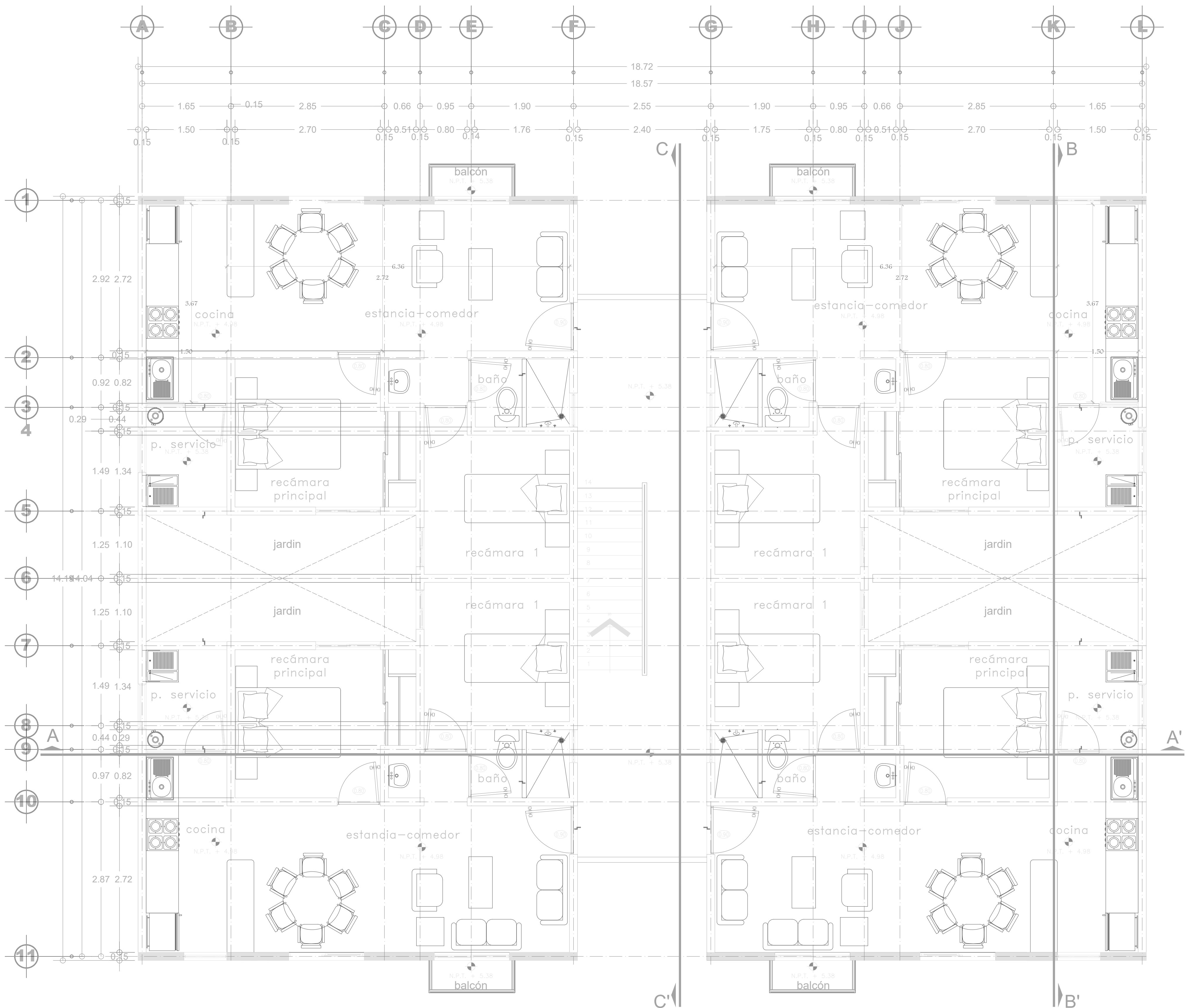
PLANTA ARQUITECTONICA 2do. NIVEL
