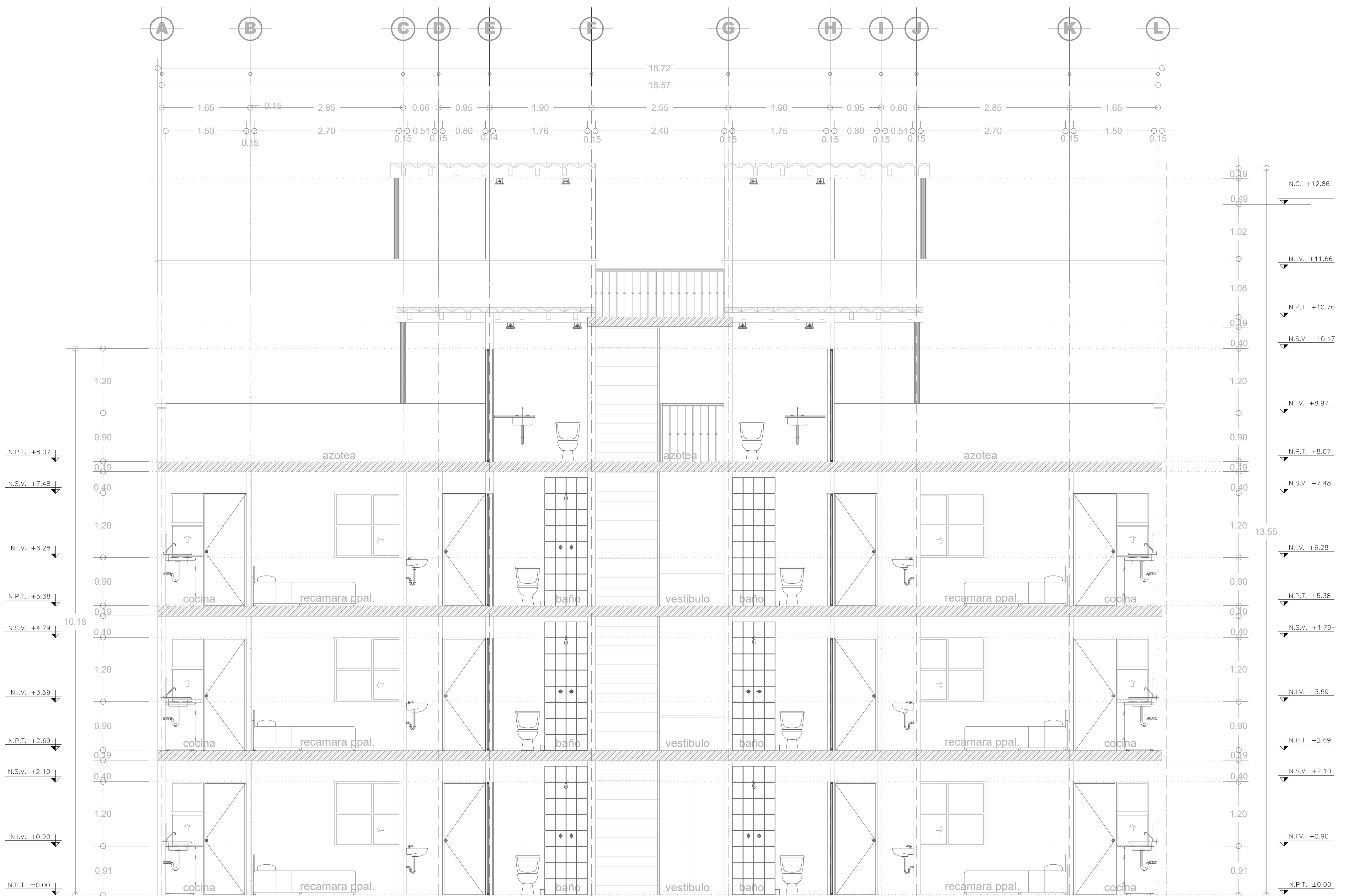
CORTE A-A'
