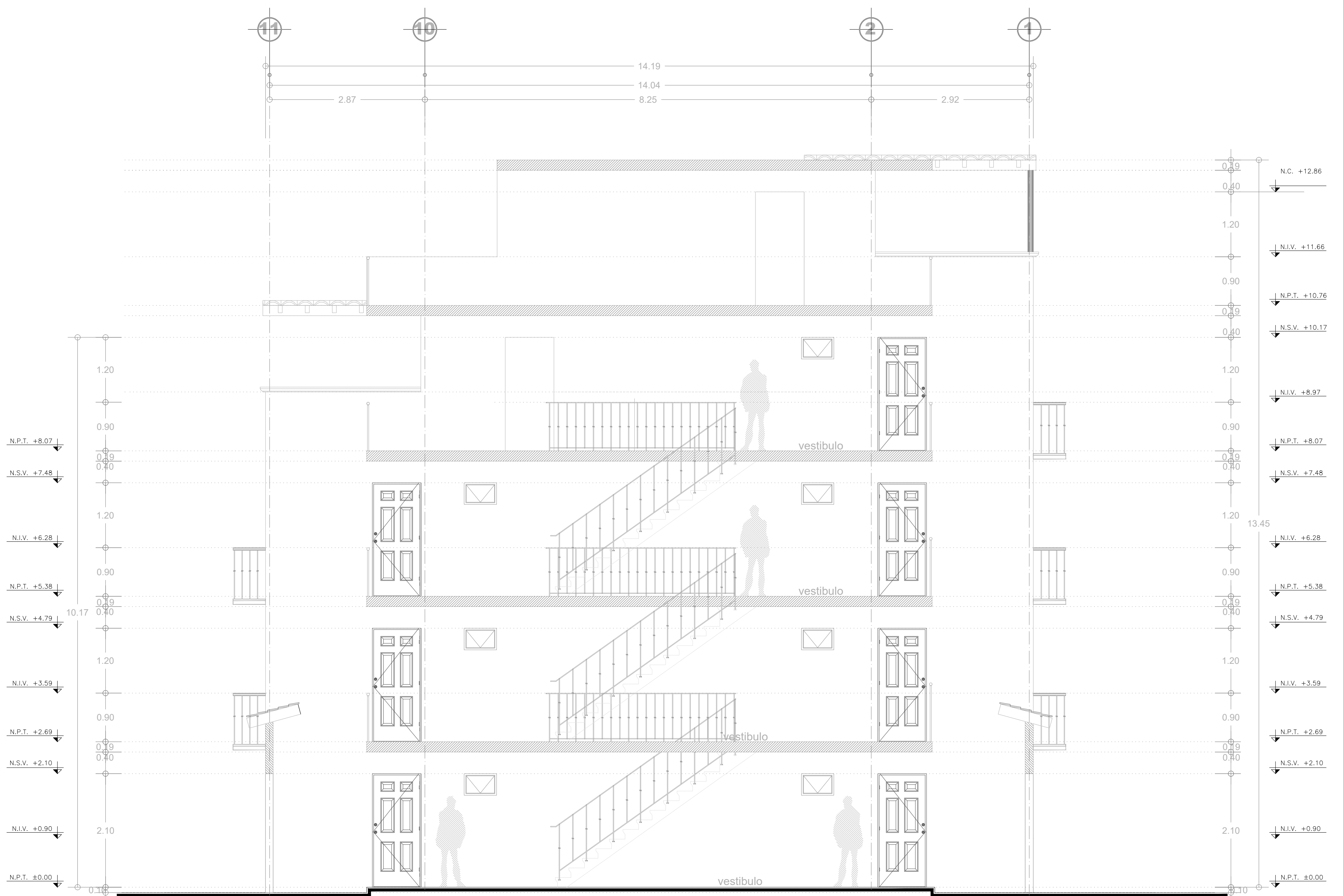
CORTE C-C'
