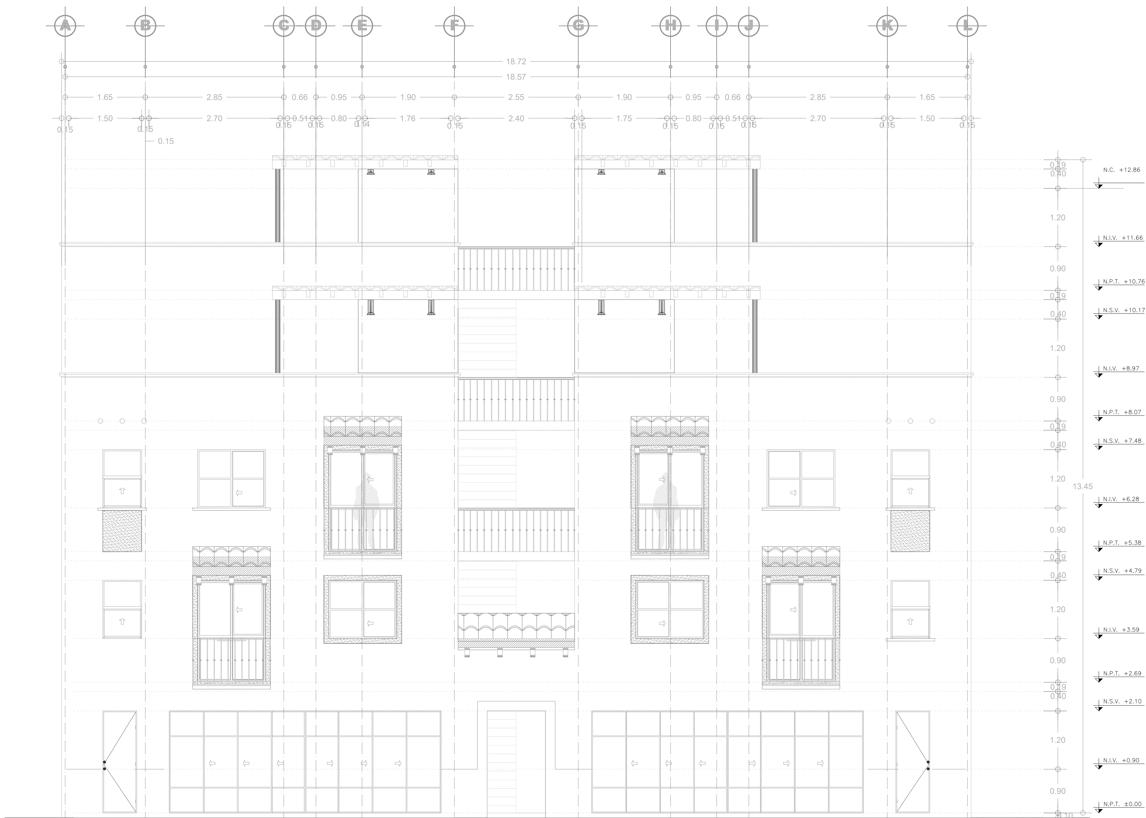
FACHADA PRINCIPAL (4 NIVELES)
