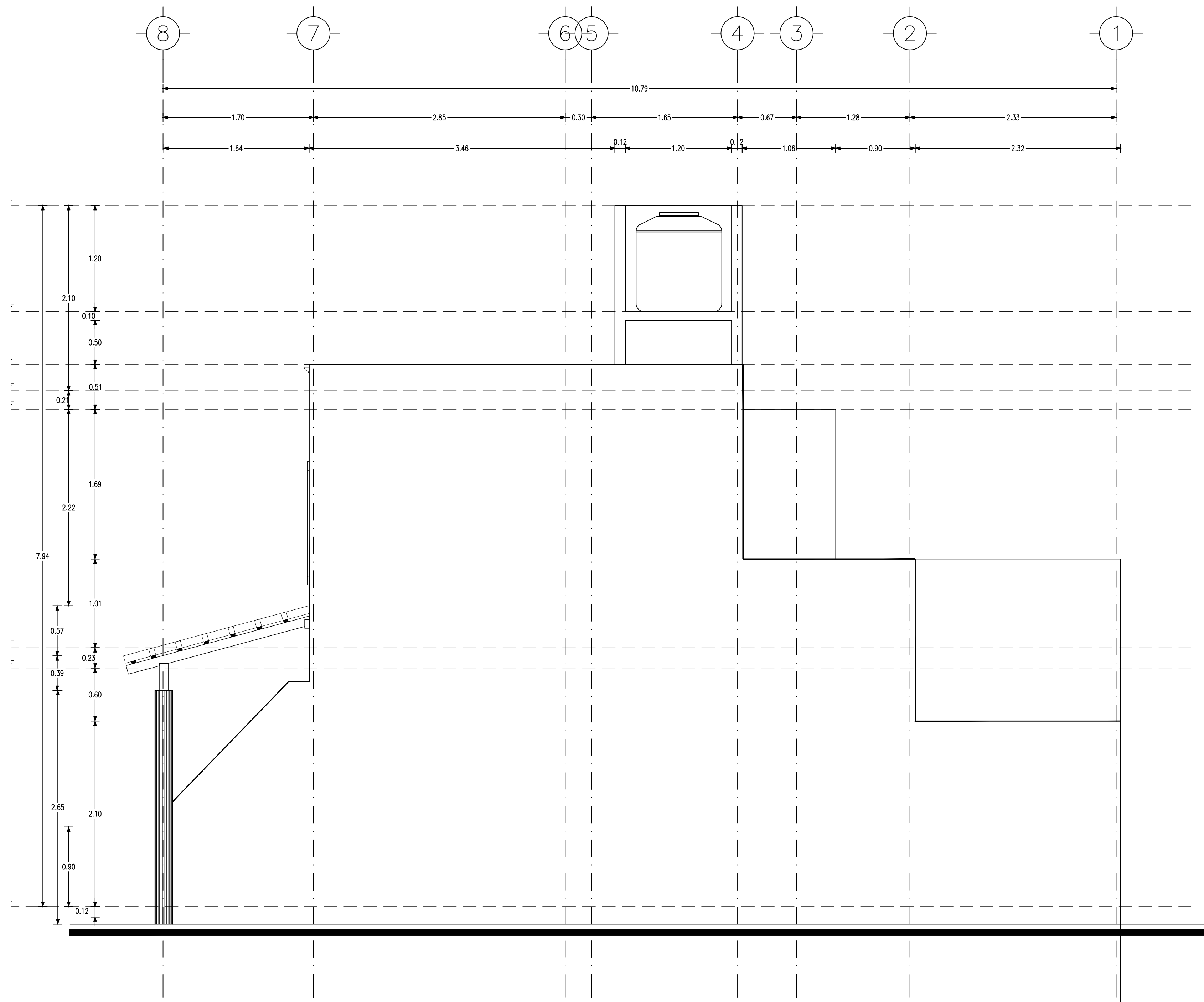
1 ARQ-04 FACHADA 02 LATERAL DERECHA ESC. 1:30 ACOT: Mts
