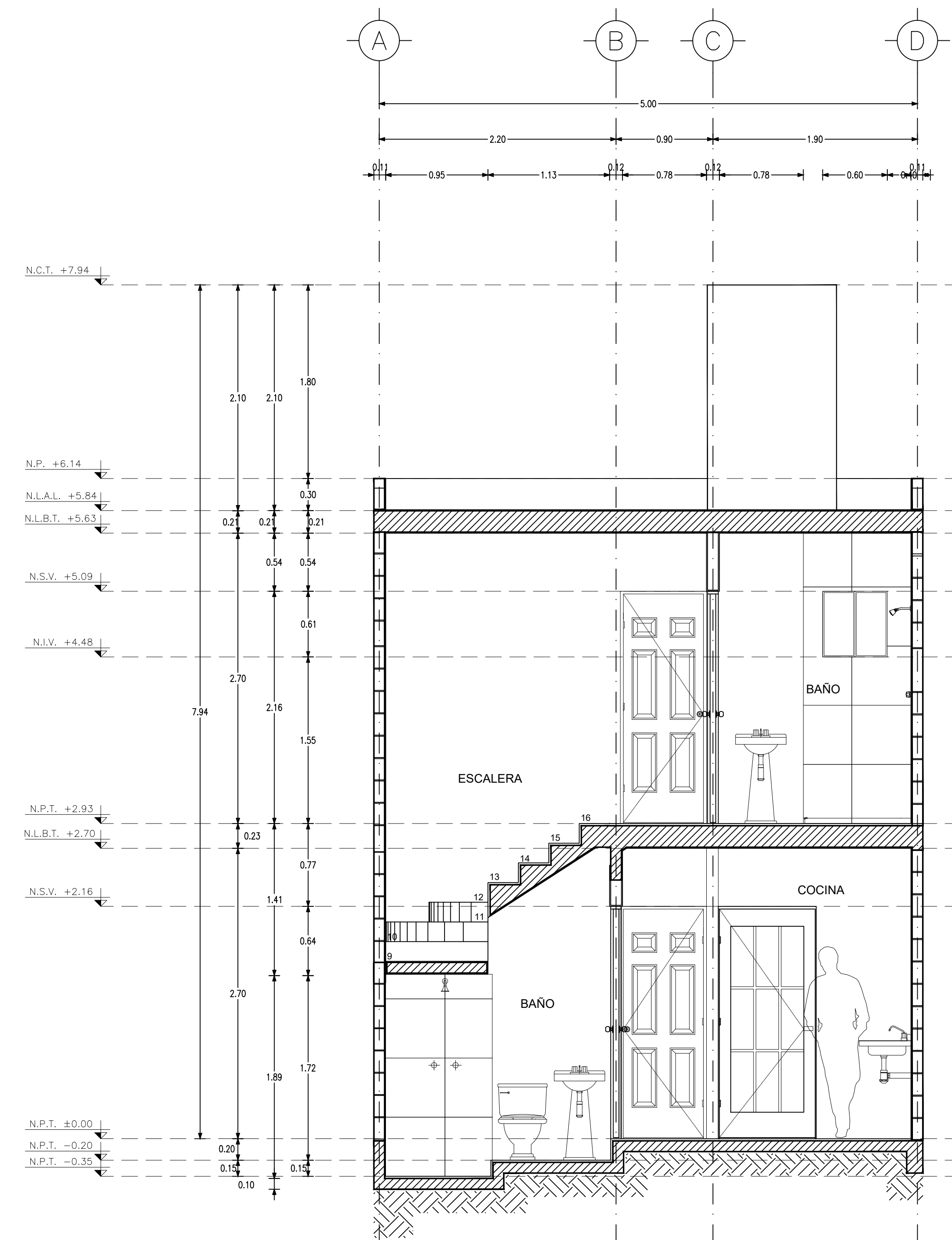
2 ARQ-04 CORTE 01 ESC. 1:30 ACOT: Mts
