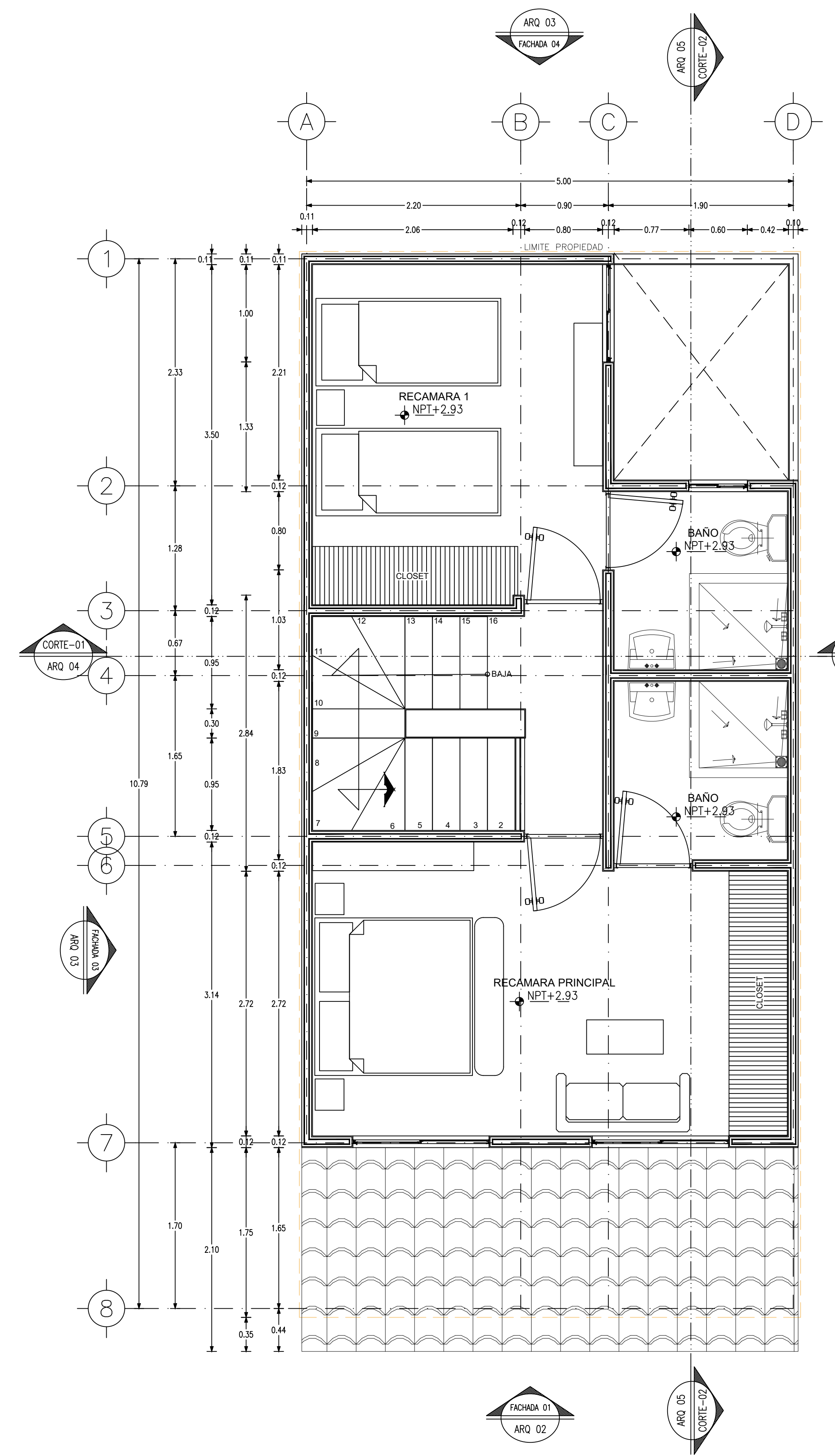
2 PLANTA ALTA ARQ-01 ESC. 1:30 ACOT: Mts
