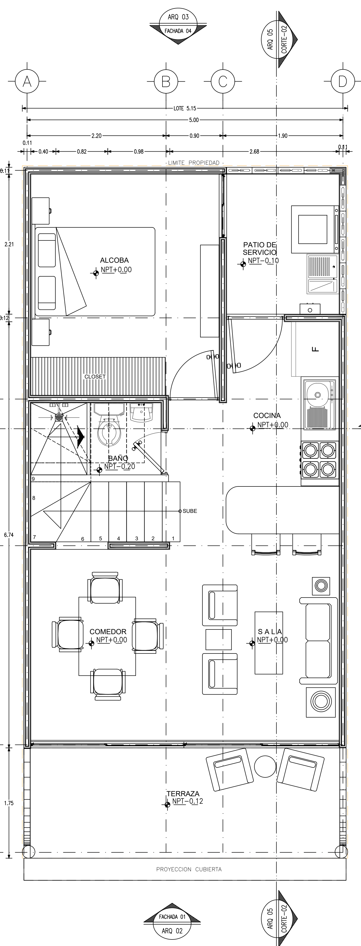
1 PLANTA BAJA ARQ-01 ESC. 1:30 ACOT: Mts
