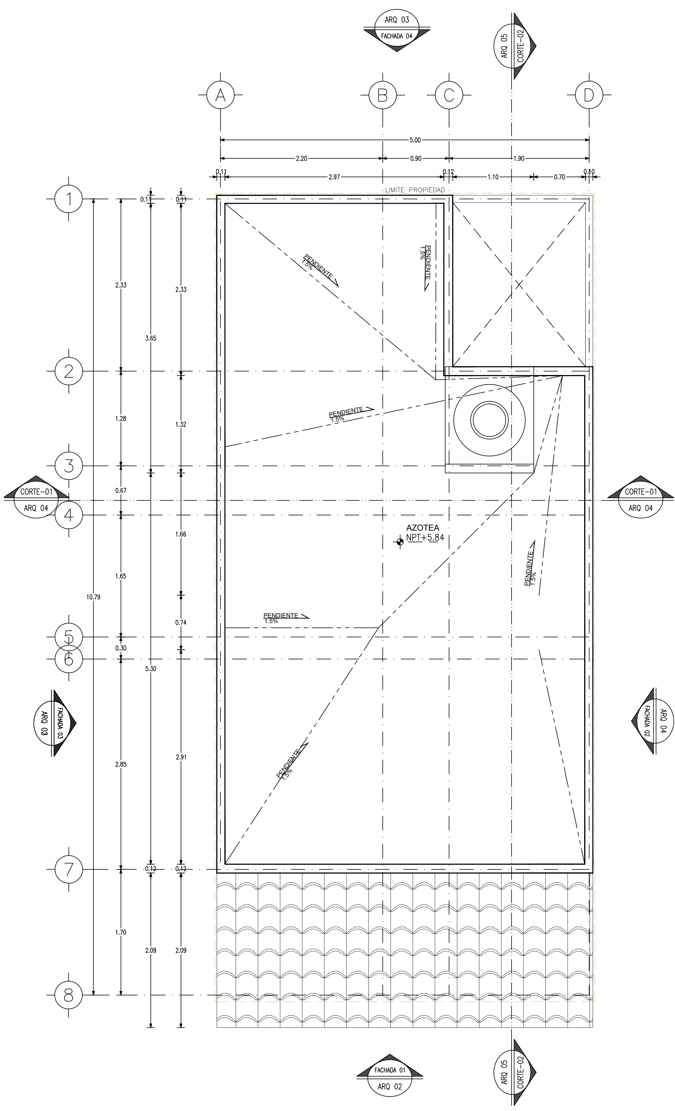
1 PLANTA AZOTEA ARQ-02 ESC. 1:30 ACOT: Mts
