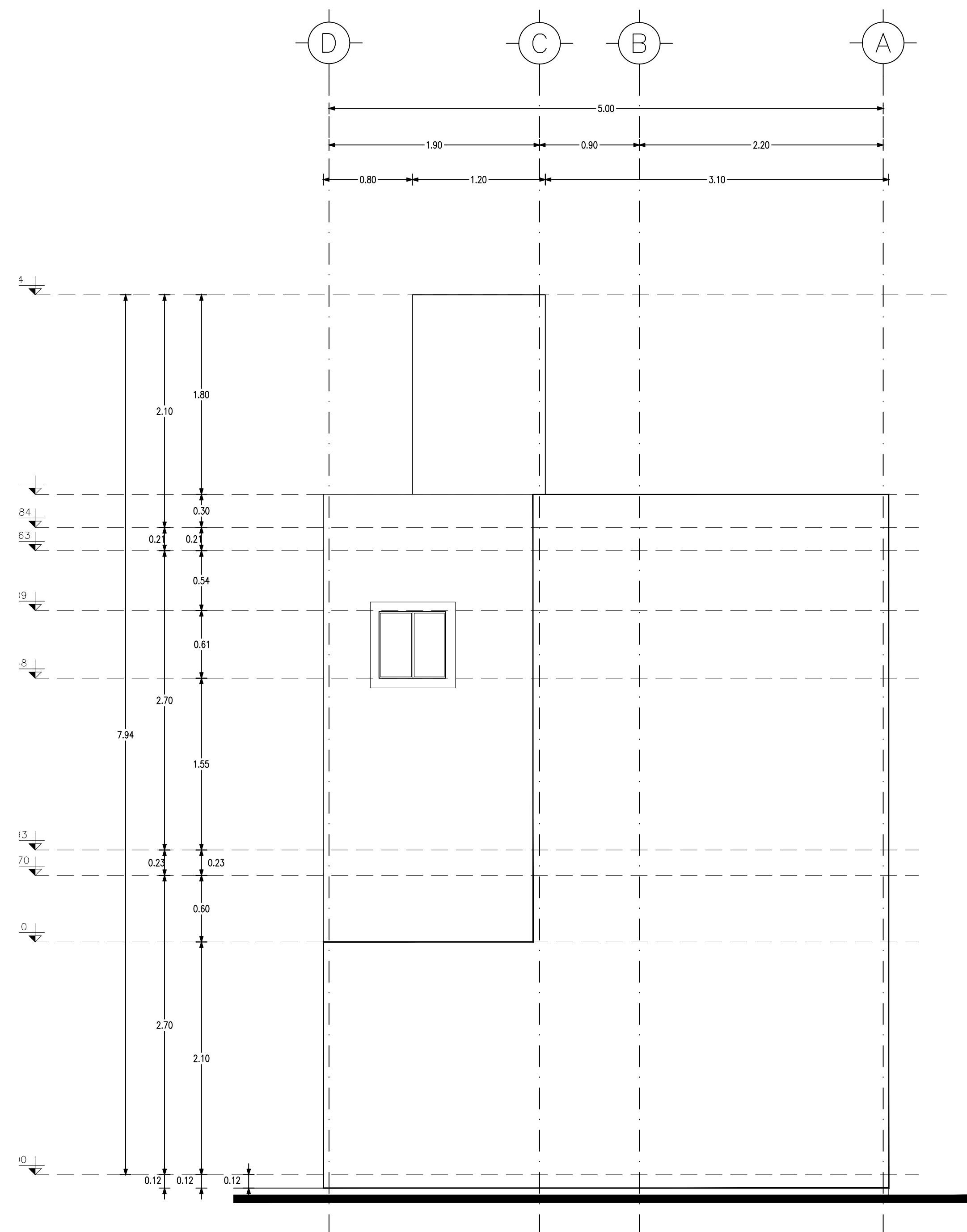
1 ARQ-03 FACHADA 04 POSTERIOR ESC. 1:30 ACOT: Mts
