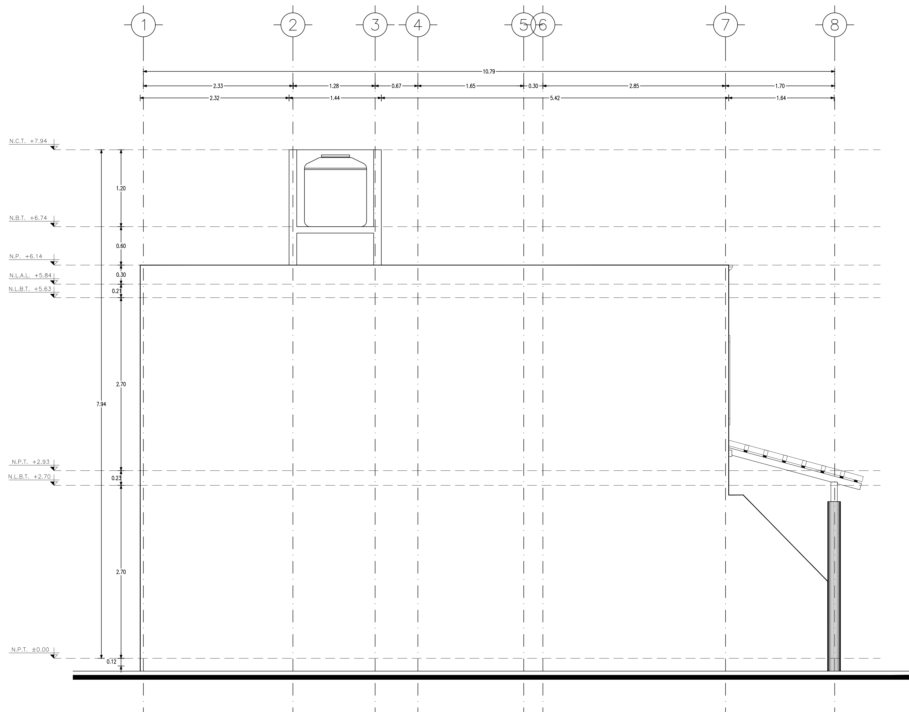
2 ARQ-03 FACHADA 03 LATERAL IZQUIERDA ESC. 1:30 ACOT: Mts
