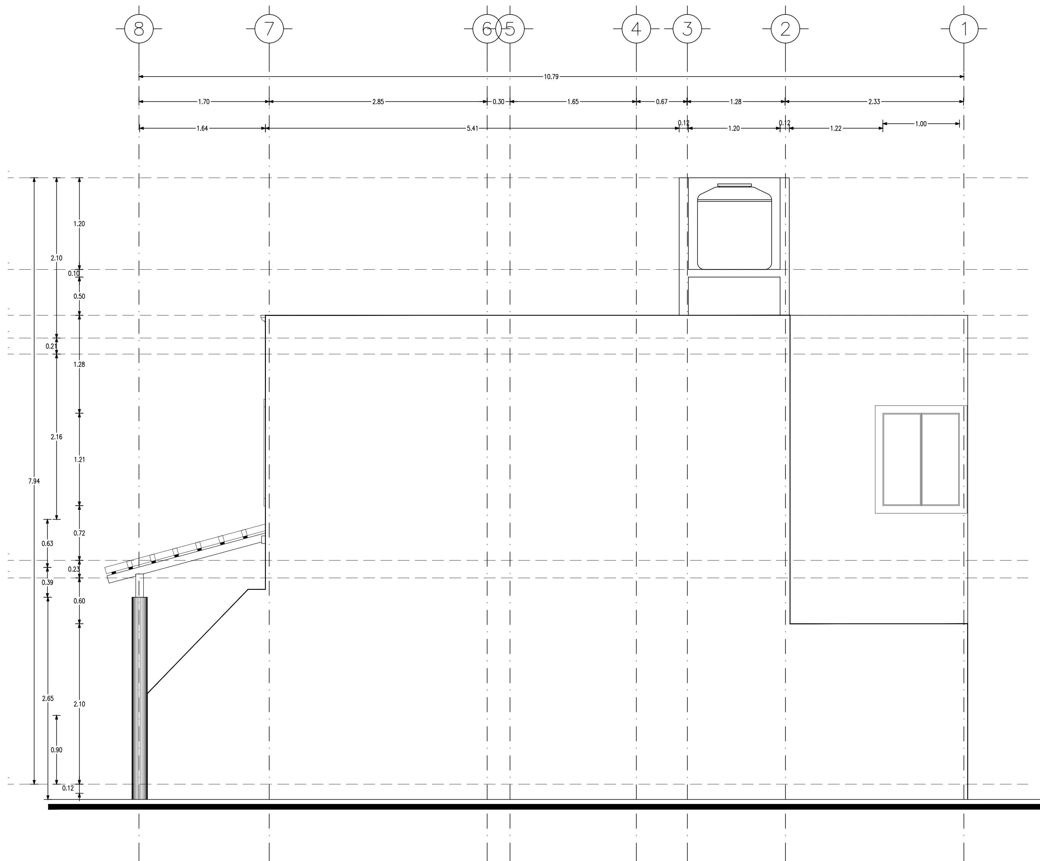
1 FACHADA 02 LATERAL DERECHA ARQ-04 ESC. 1:30 ACOT: Mts
