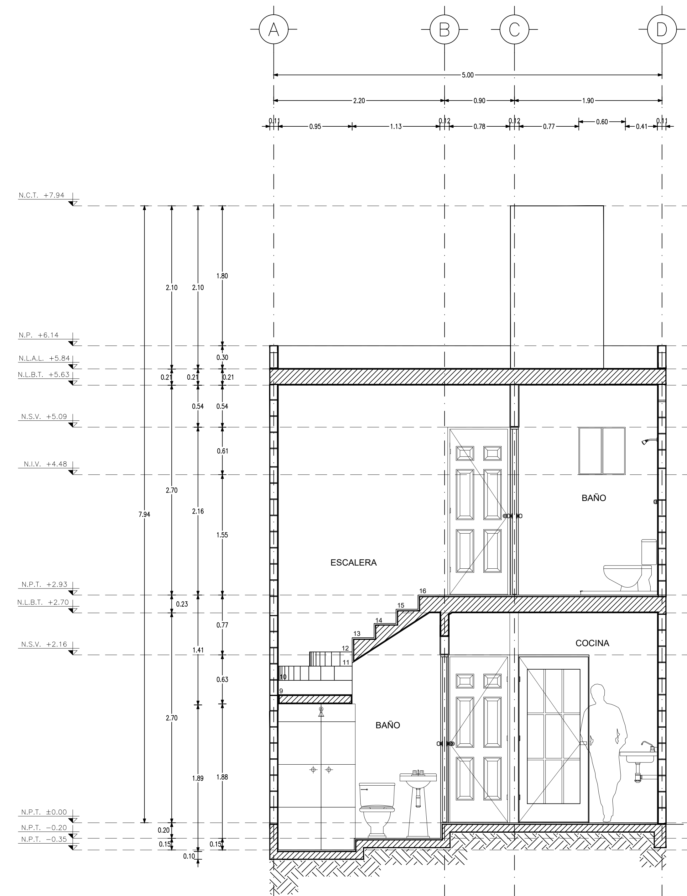
2 CORTE 01 ARQ-04 ESC. 1:30 ACOT: Mts
