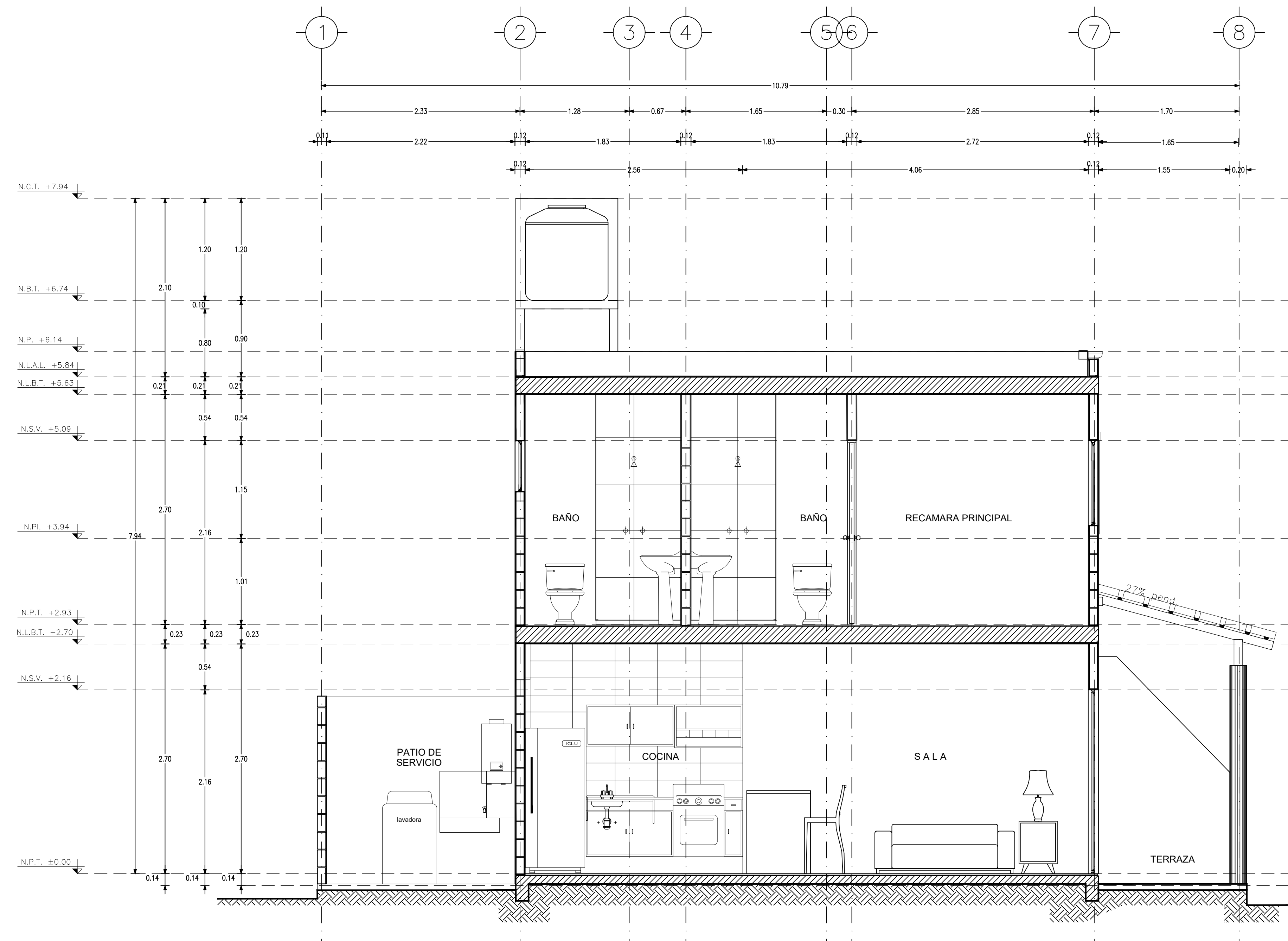
1 ARQ-05 CORTE 02 ESC. 1:30 ACOT: Mts
